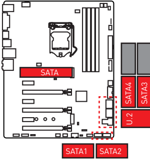
1xM.2 SATA+ 1xU.2+ 4xSATA
