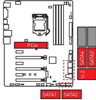
1xM.2 PCIe+ 1xU.2+ 4xSATA
